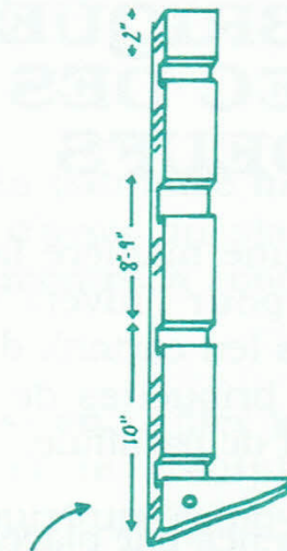
Position des traverses sur les montants
