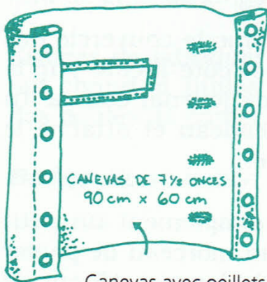
Canevas avec oeillets et ouverture
